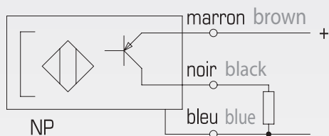
Détecteur magnétique type DM1 Magnetic sensor type DM1
